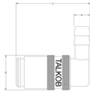
Schnellverschlusskupplung mit Tülle gewinkelt 90°
