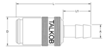
Schnellverschlusskupplung mit Tülle
