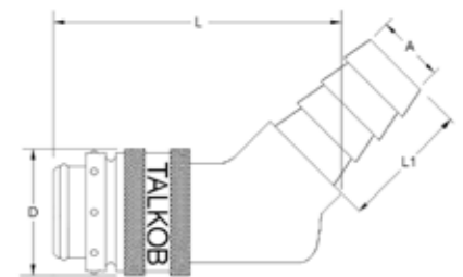
Schnellverschlusskupplung mit Tülle gewinkelt 45°
