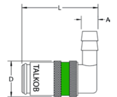
Schnellverschlusskupplung mit Tülle und Automatischem Verschluss - gewinkelt 90° SAFE LOCK
