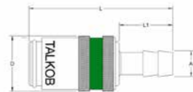
Schnellverschlusskupplung mit Tülle und automatischem Verschluss - SAFE LOCK
