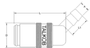
Schnellverschlusskupplung mit Tülle gewinkelt 45°
