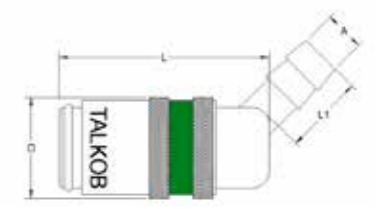
Schnellverschlusskupplung mit Tülle und Automatischem Verschluss - gewinkelt 45° SAFE LOCK
