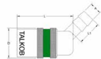
Schnellverschlusskupplung mit Tülle und Automatischem Verschluss - gewinkelt 45° SAFE LOCK
