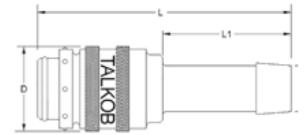
Schnellverschlusskupplung mit Tülle
